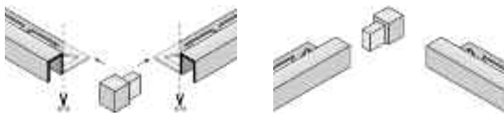
Růžek Y pro vnější i vnitřní roh
